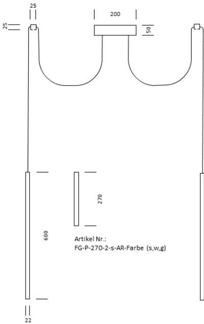
2er Pendelleuchte Freigeist mit Baldachin Aufbau rund und Deckenabnehmer Artikel Nr.: FG-P-600-2-s-AR-Farbe (s,w,g)
